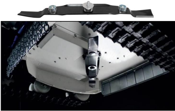
CUCHILLAS FLOTANTES (X-ROT 70, 70 PRO, 80 PRO y 95)
